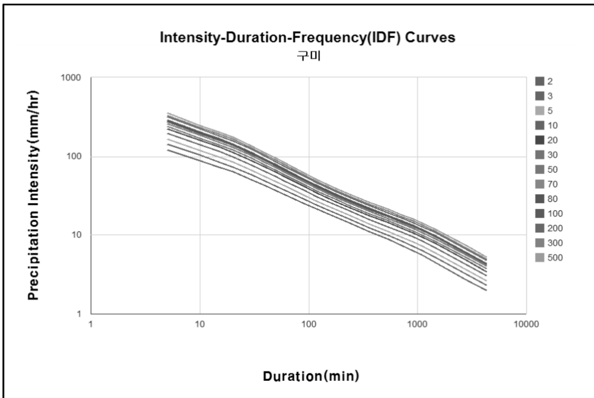
【그림 5.9】 구미지역 IDF곡선
