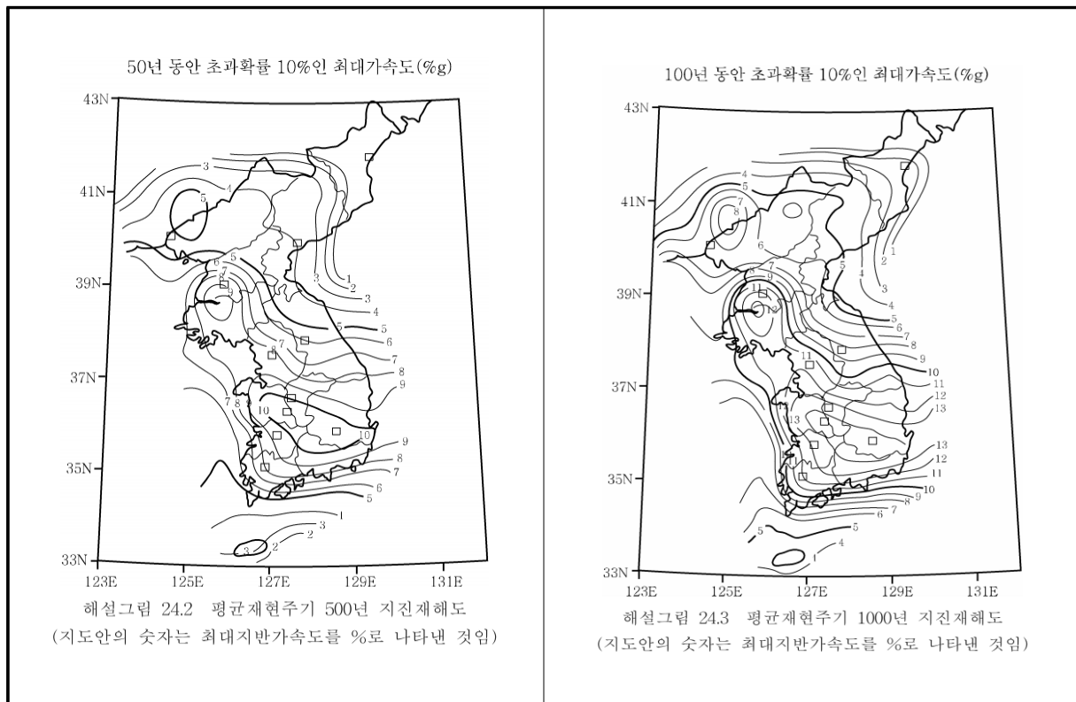
【그림 5.12】 평균재현주기 500년 및 1000년 지진재해도
