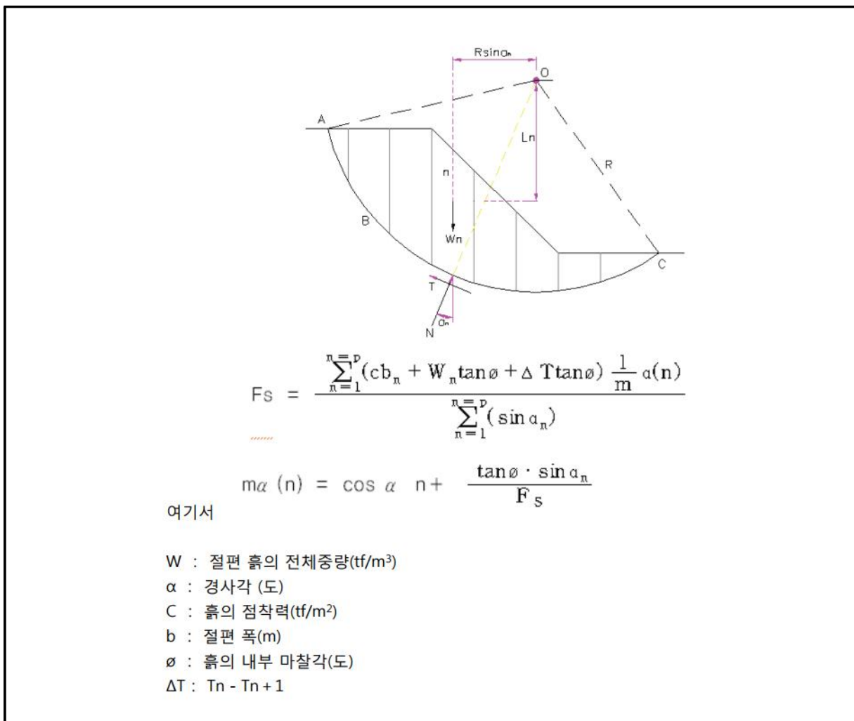
【그림 5.7】 Bishop의 안전율 계산식
