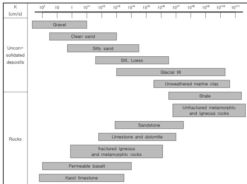
【그림 5.8】 퇴적물 및 암종별 투수계수(Freeze &amp; Cherry, 1979)
